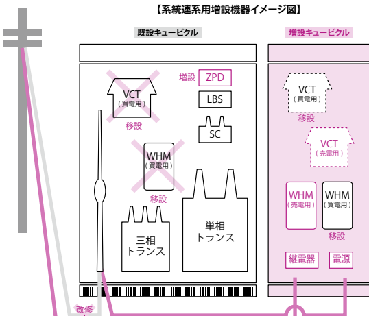
【系統連系用増設機器イメージ図】
