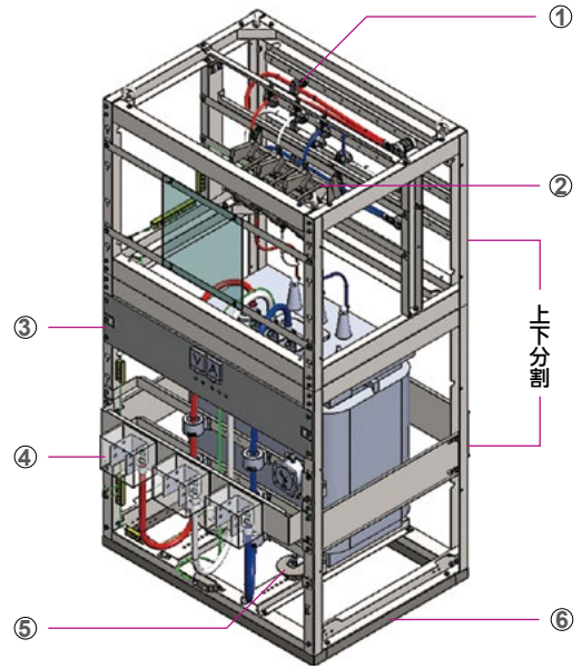
トランス盤 上下2分割仕様 適応トランス:1φ10kVA~300kVA 3φ20kVA~300kVA
