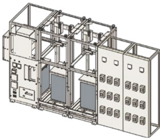
横一列配置
