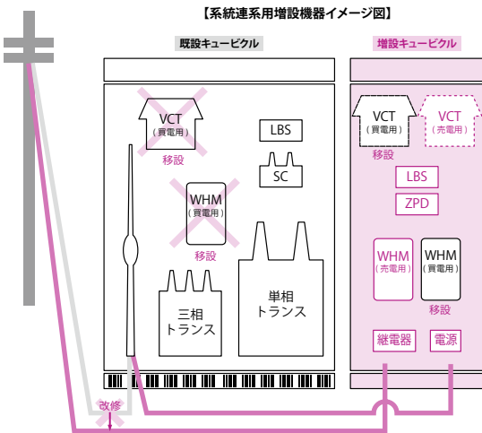
【系統連系用増設機器イメージ図】
