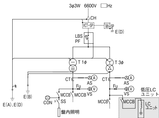
結線図(参考)
