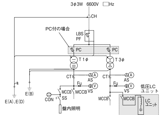
結線図(参考)
