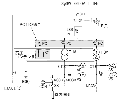
結線図(参考)
