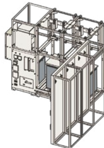
L字配置
