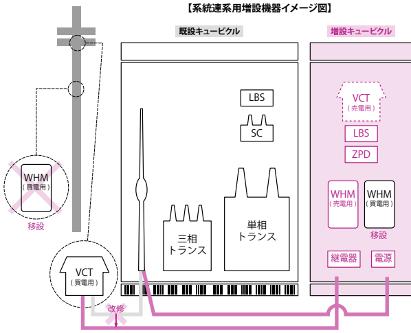
【系統連系用増設機器イメージ図】
