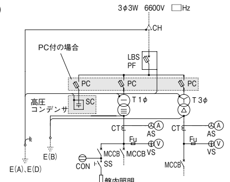
結線図(参考)
