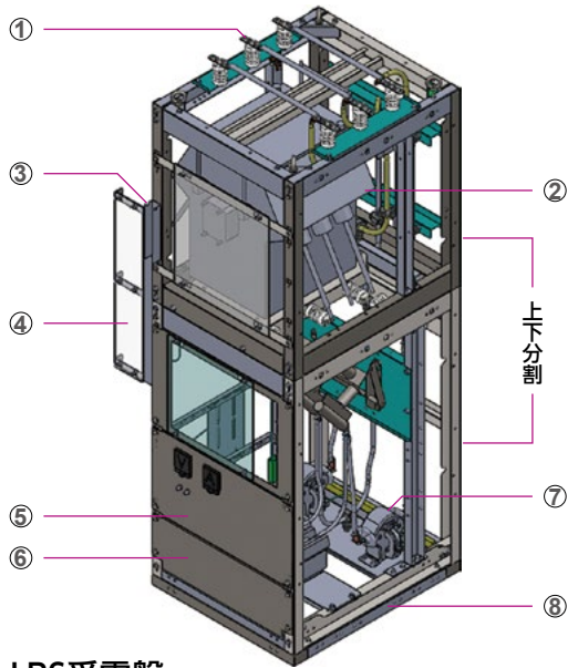
LBS受電盤 上下2分割のコンパクトサイズ
