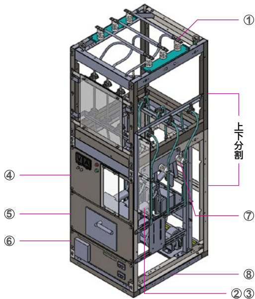
VCBき電盤 上下2分割のコンパクトサイズ
