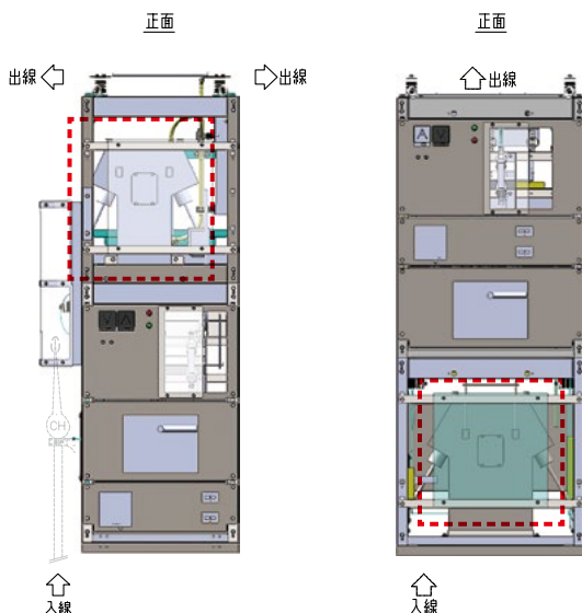
VCT上段設置型 列盤可能構造
