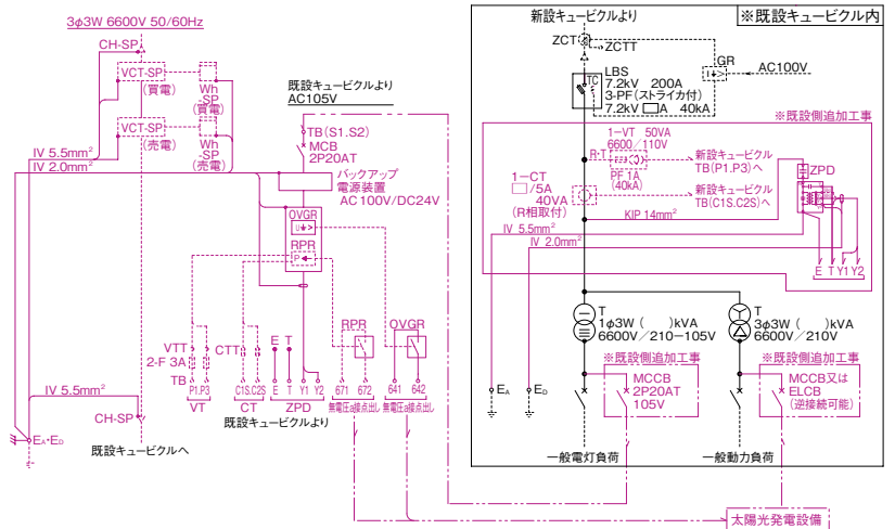
【結線図(系統連系キュービクル<増設用>)]
