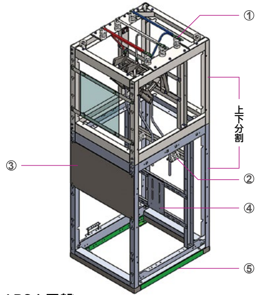
LBSき電盤 上下2分割のコンパクトサイズ
